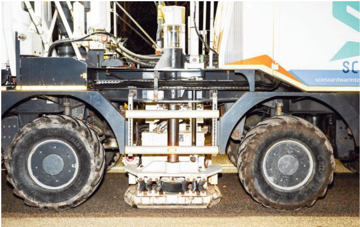
Een plaat (hier-naast) onder een vrachtauto stuurt trillingen de grond in die door kastjes (midden) worden geregistreerd. Een app (boven) laat zien waar de auto al is geweest.
