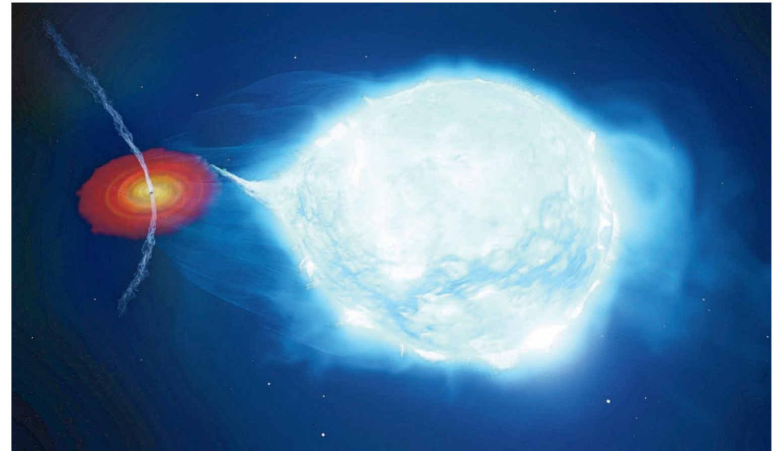
Dubbelstersysteem Cygnus X-1 voedt het zwarte gat en blaast de relativistische jets van het zwarte gat opzij. ILLUSTRATIE ICRAR
